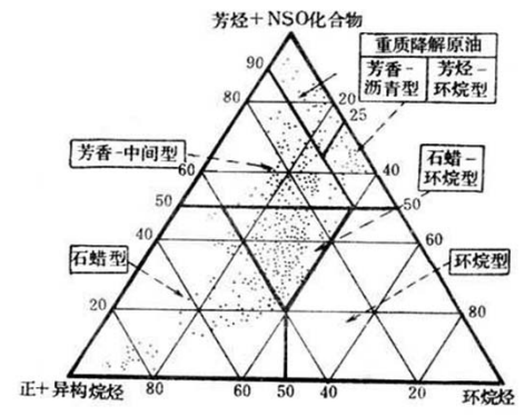
图1 6种原油类型的三角图解
